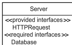
Gráfico 2: Interfaces en el compartimiento de un clasifi. Tomado de Ivers y otros (2004)
