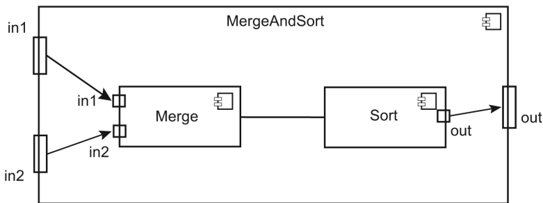
Gráfico 7: Un componente estructurado en UML 2.0. Tomado de Ivers y otros (2004)
